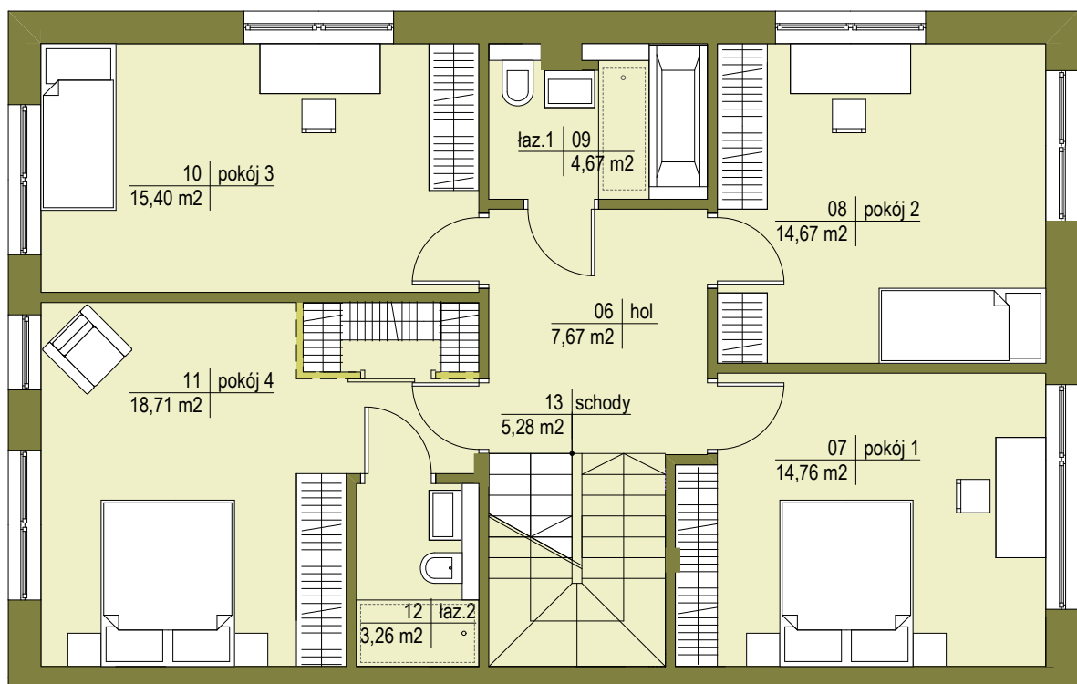
PIĘTRO
