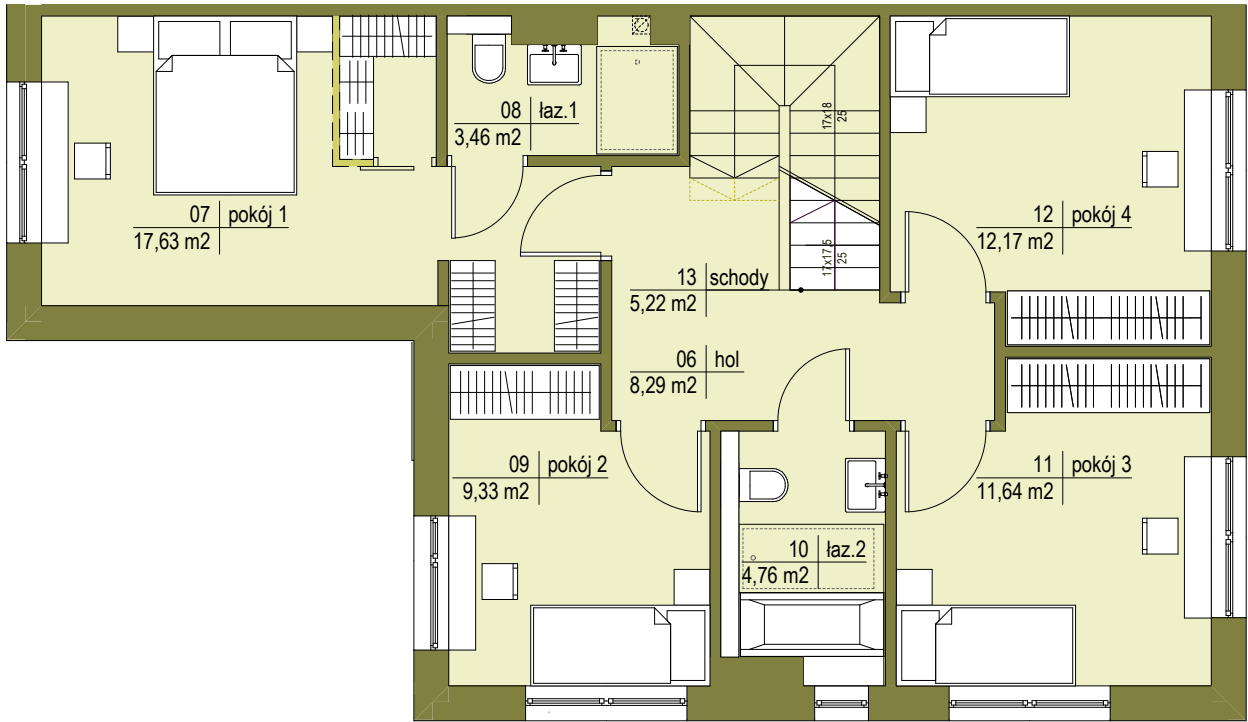
PIĘTRO
