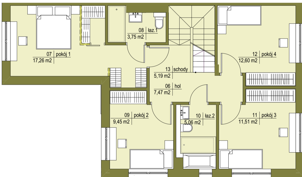
PIĘTRO
